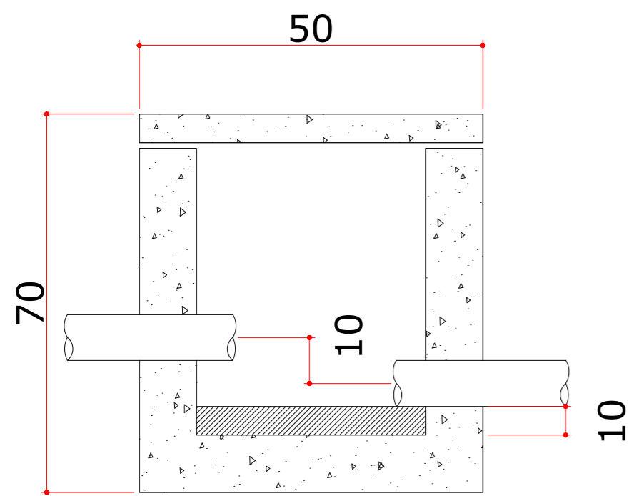
CORTE TRANSVERSAL CAIXA DE AREIA sem escala
