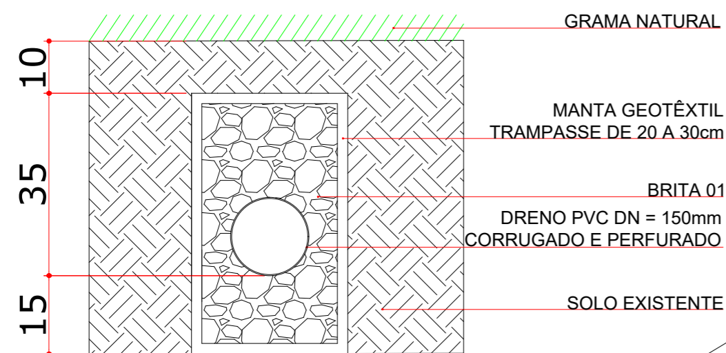
CORTE TRANSVERSAL DRENO BRITA sem escala
